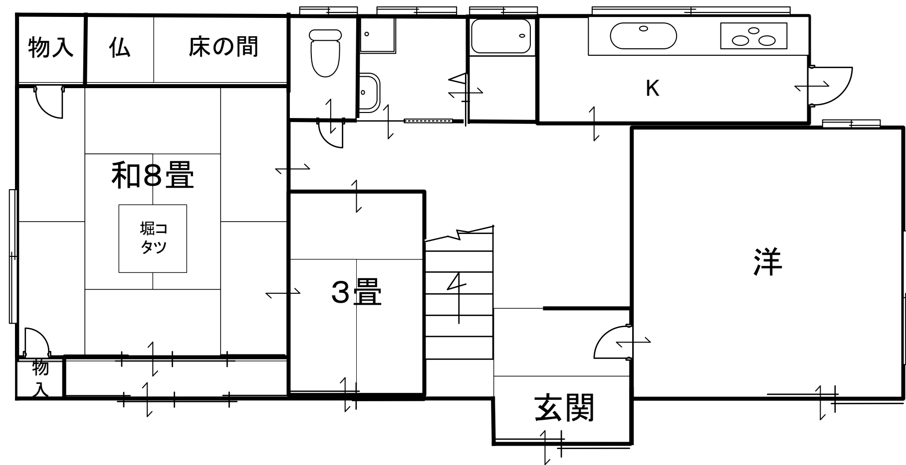
【1F】
